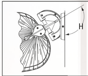
PUNKAH bestehend aus PUNKAH Motor PW #FP780PW Gehäuse und Metallteile Zinn, 5 Stück Flügelbasis PUNKAH Flügelbasis PW #FP720PW Metallteile Zinn und 5 Stück Flügel Palme natur, #PUP1
